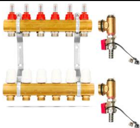
Rozdělovač s uzavíracími ventily a regulačním šroubením s průtokoměry pro podlahové vytápění, připojení G1", výstup pro svěrné šroubení G3/4" s eurokonusem.
